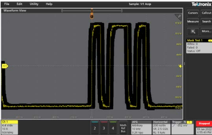
골든 참조 신호를 기준으로 마스크 테스트를 제한
