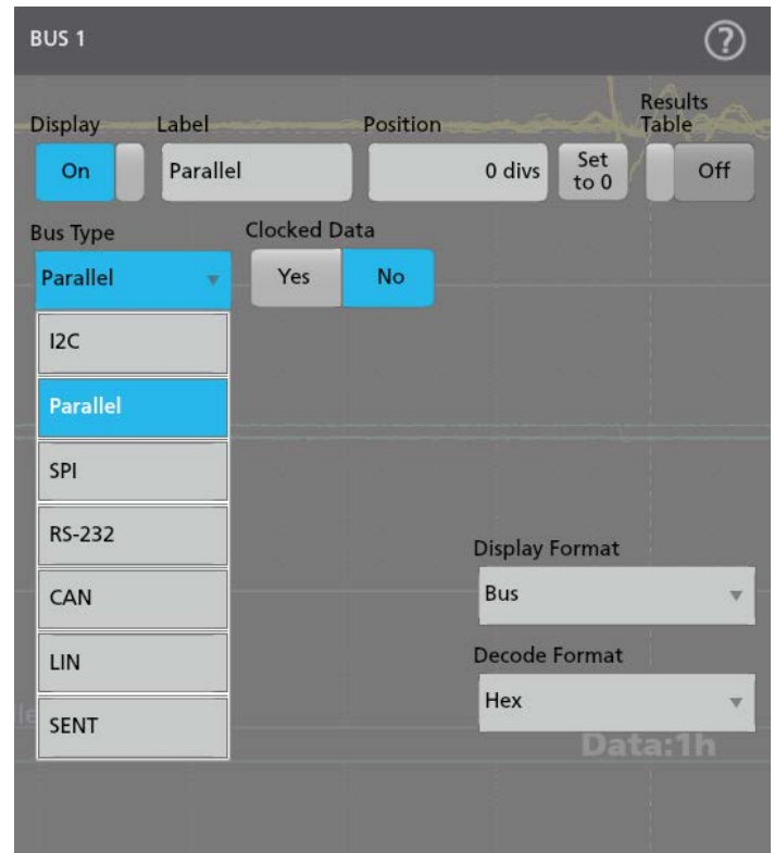
버스 메뉴는 버스 매개변수를 구성하는 옵션 제공
